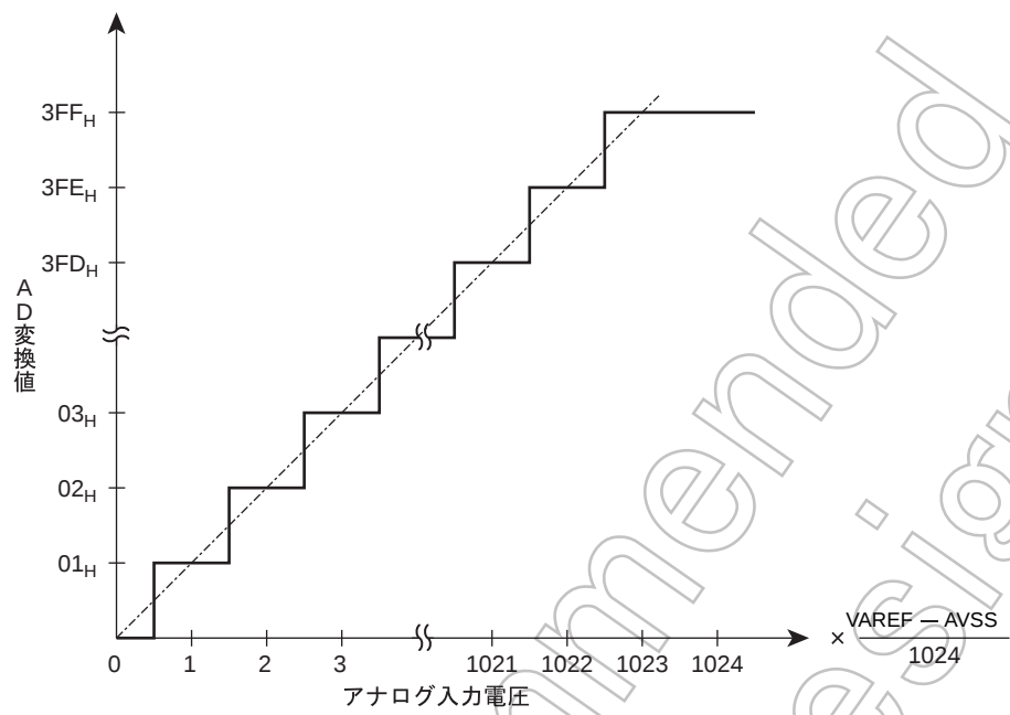
図 15-4 アナログ入力電圧と AD 変換値 (typ.) の関係
