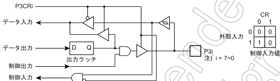
図 5-4 P3 ポート
