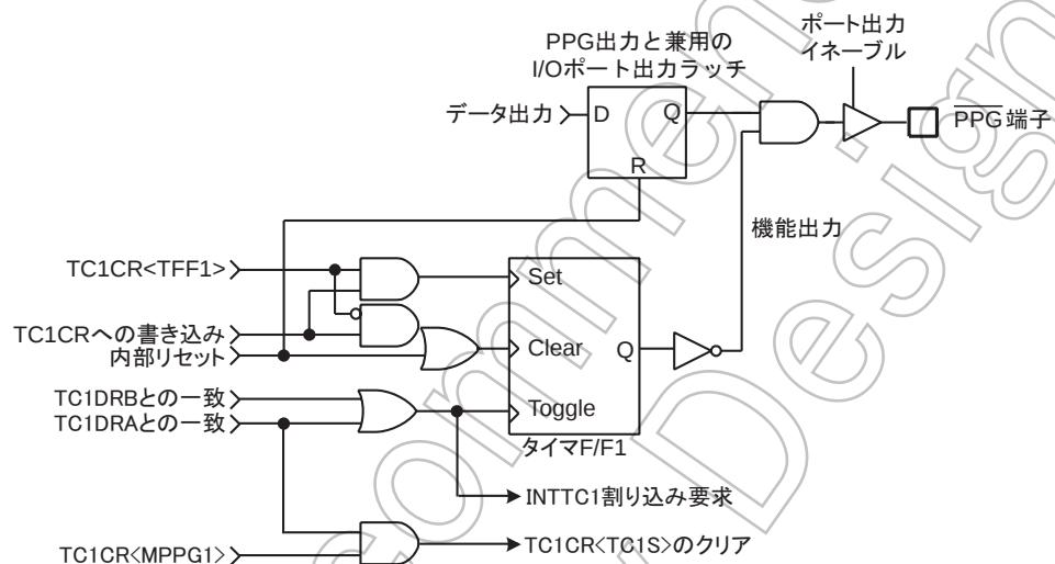
図 8-7 \overline{\text{PPG}} 出力
