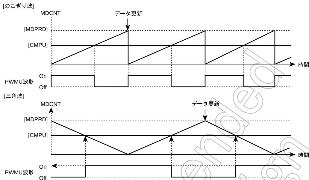
図 12-9 PWM 波形
