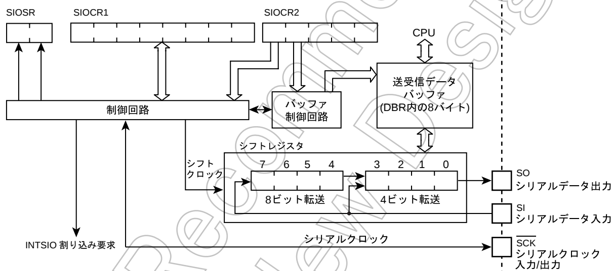
図 14-1 シリアルインタフェース
