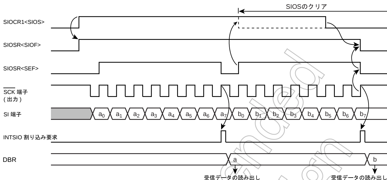
図 14-10 受信モード (例: 8 ビット, 1 ワード転送, 内部クロック)
