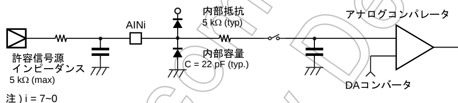
図 15-5 アナログ入力等価回路と入力端子処理例
