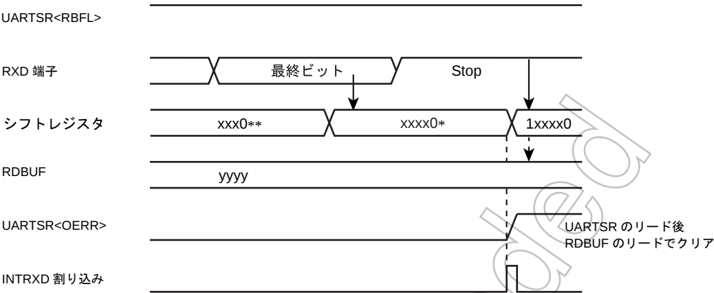
図 13-7 オーバランエラーの発生
