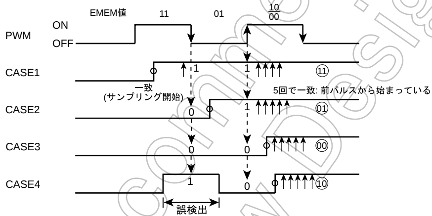
図 12-6 位置検出位置の検出タイミング
