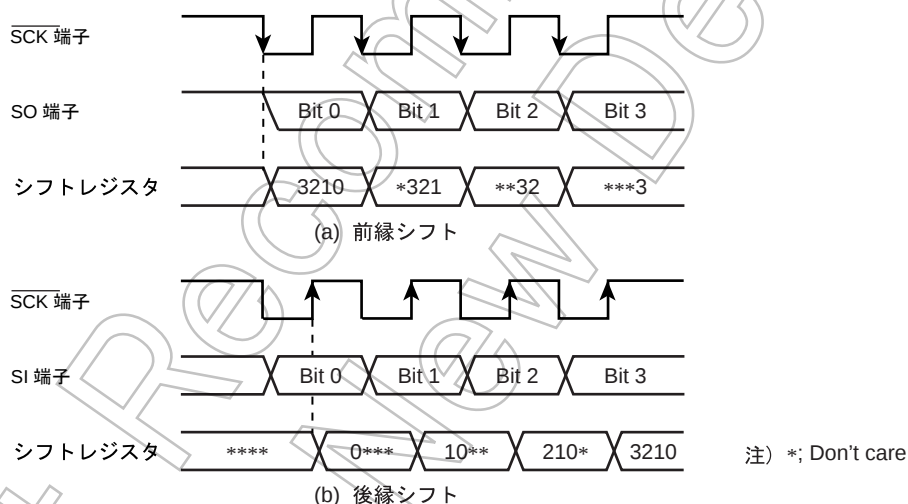
図 14-5 シフトエッジ
