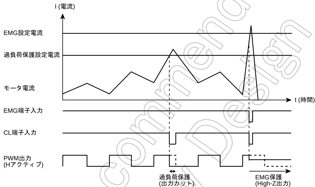
図 12-14 保護回路動作例
