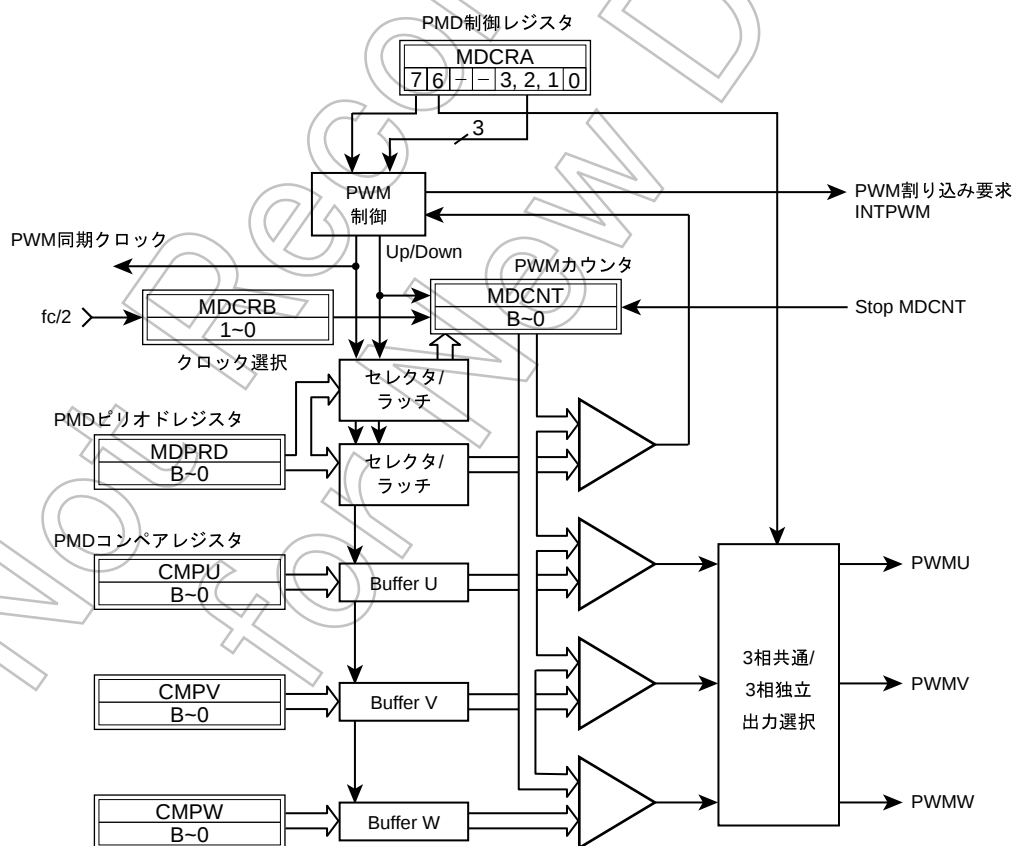
図 12-10 パルス幅変調回路
