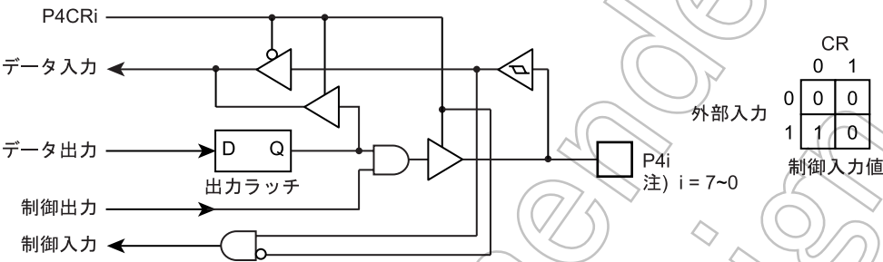
図 5-5 P4 ポート
