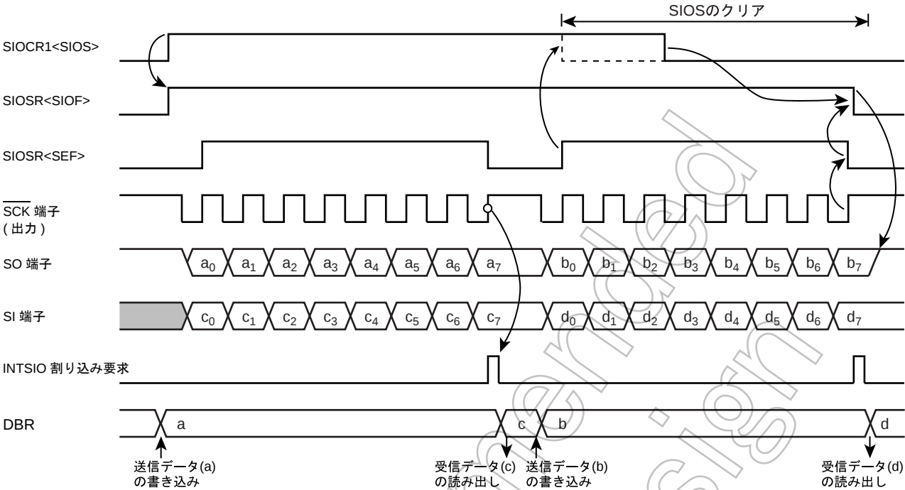
図 14-11 送受信モード (例 : 8 ビット , 1 ワード , 内部クロック)
