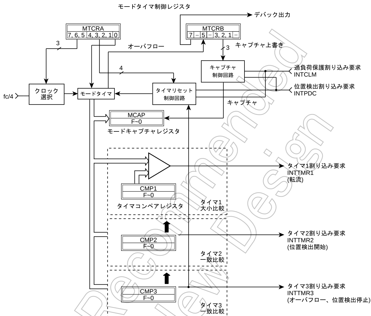
図 12-7 タイマ回路構成
