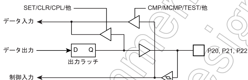
図 5-3 P2 ポート
