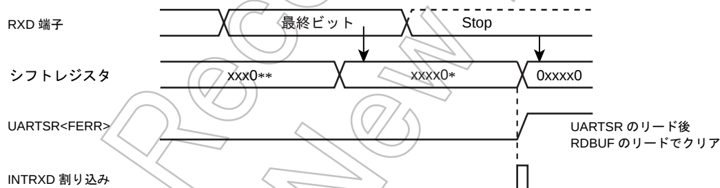
図 13-6 フレーミングエラーの発生
