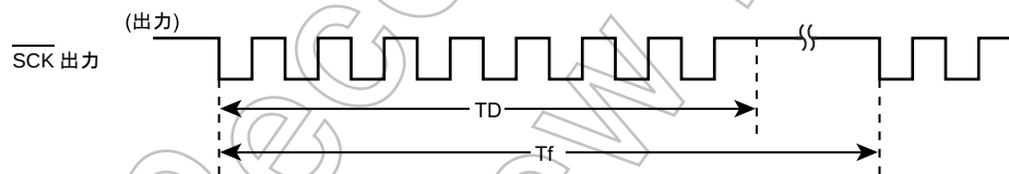
図 14-2 フレーム時間 ( T_f ) とデータ転送時間 ( T_D )
