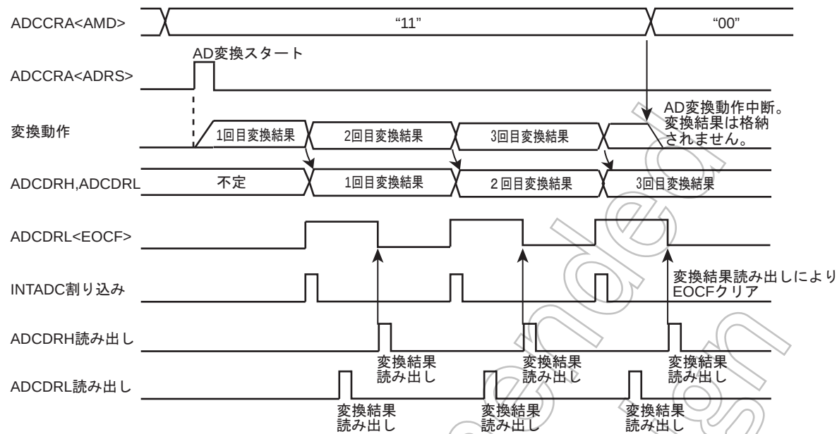
図 15-3 リピートモード
