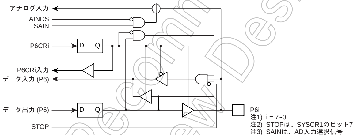
図 5-6 P6 ポート
