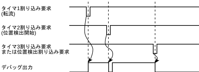
図 12-8 DBOUT デバッグ出力図
