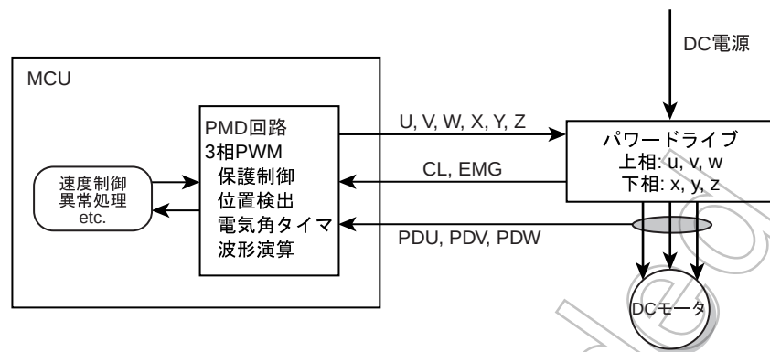
図 12-1 DC モータ制御概念図
