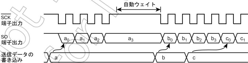
図 14-3 自動ウェイト機能 (4 ビット送信モードの場合)
