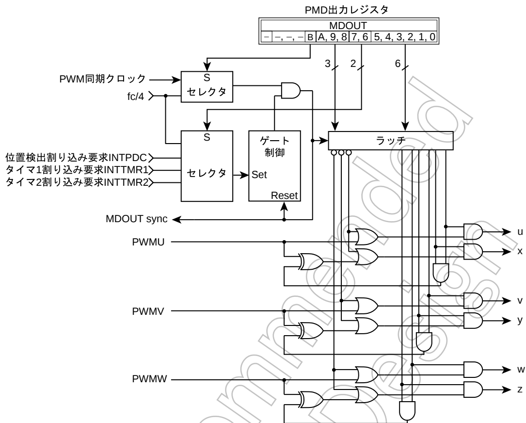
図 12-11 転流制御回路
