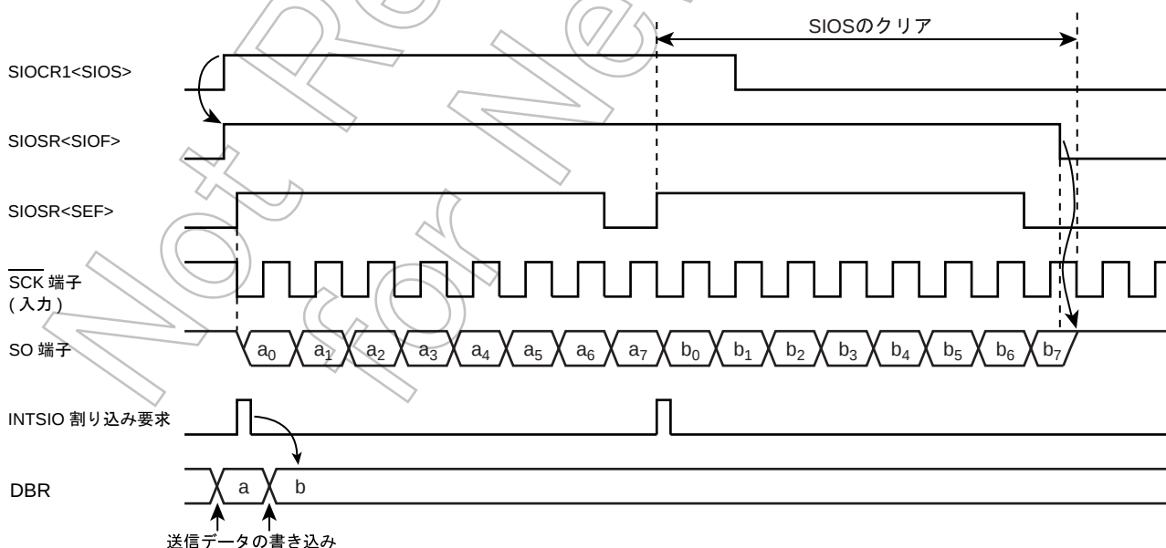
図 14-8 送信モード (例: 8 ビット, 1 ワード転送、外部クロック)
