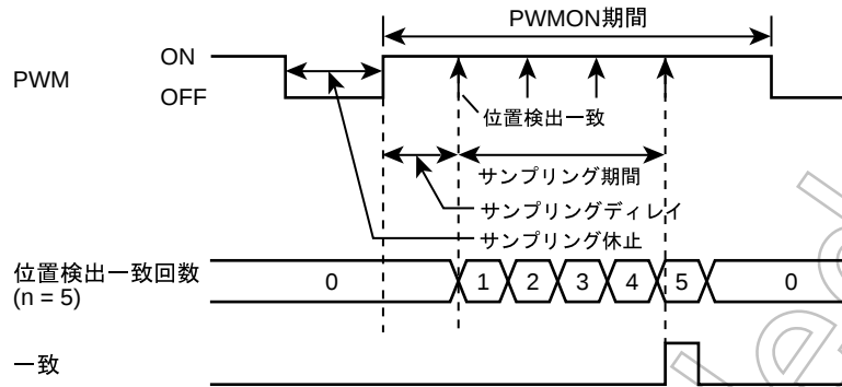
図 12-5 PWMON 時選択時の位置検出サンプリングタイミング
