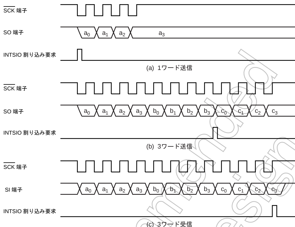
図 14-6 転送ワード数 (例 : 1 ワード = 4 ビット)
