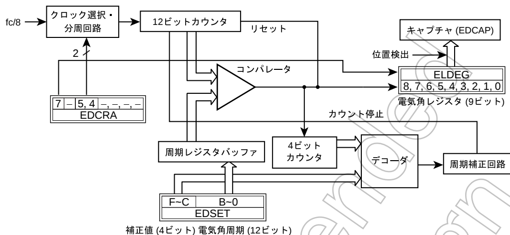
図 12-15 電気角タイマ回路
