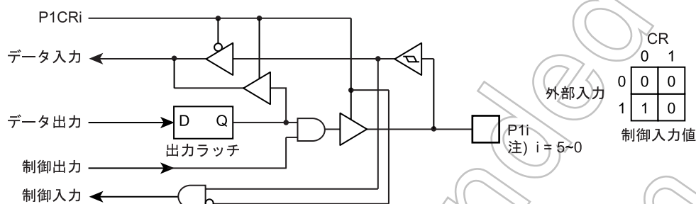
図 5-2 P1 ポート
