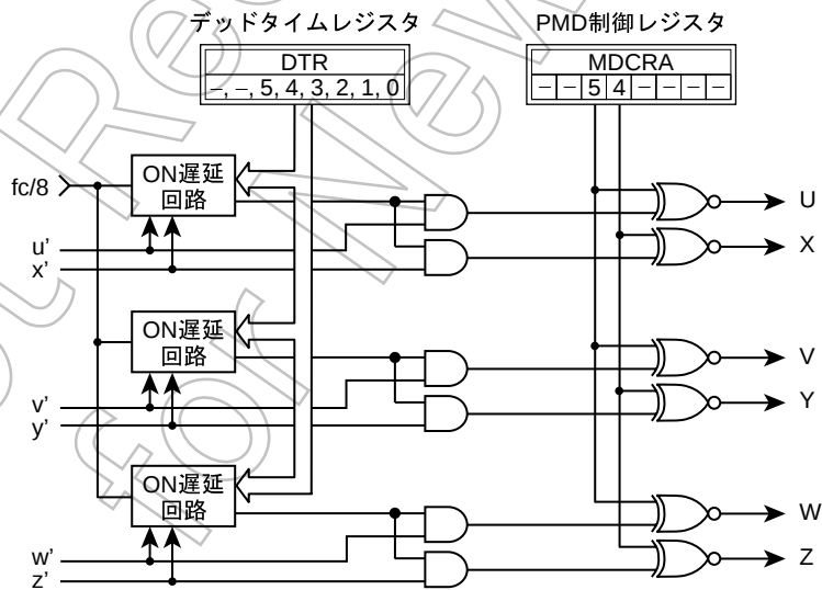
図 12-12 デッドタイム回路
