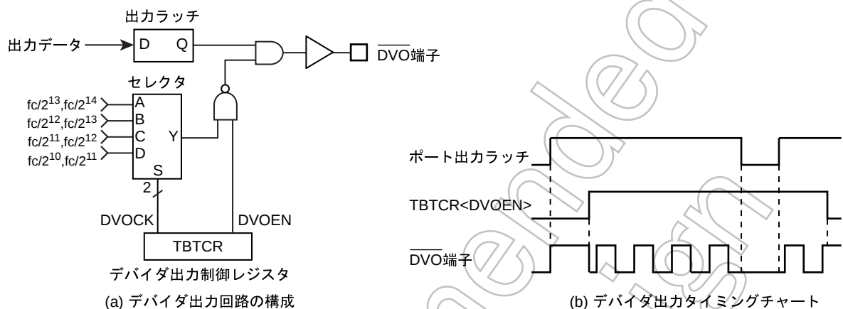
図 7-2 デバイダ出力
