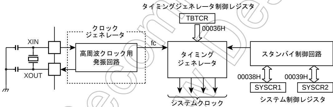
図 2-2 システムクロック制御回路
