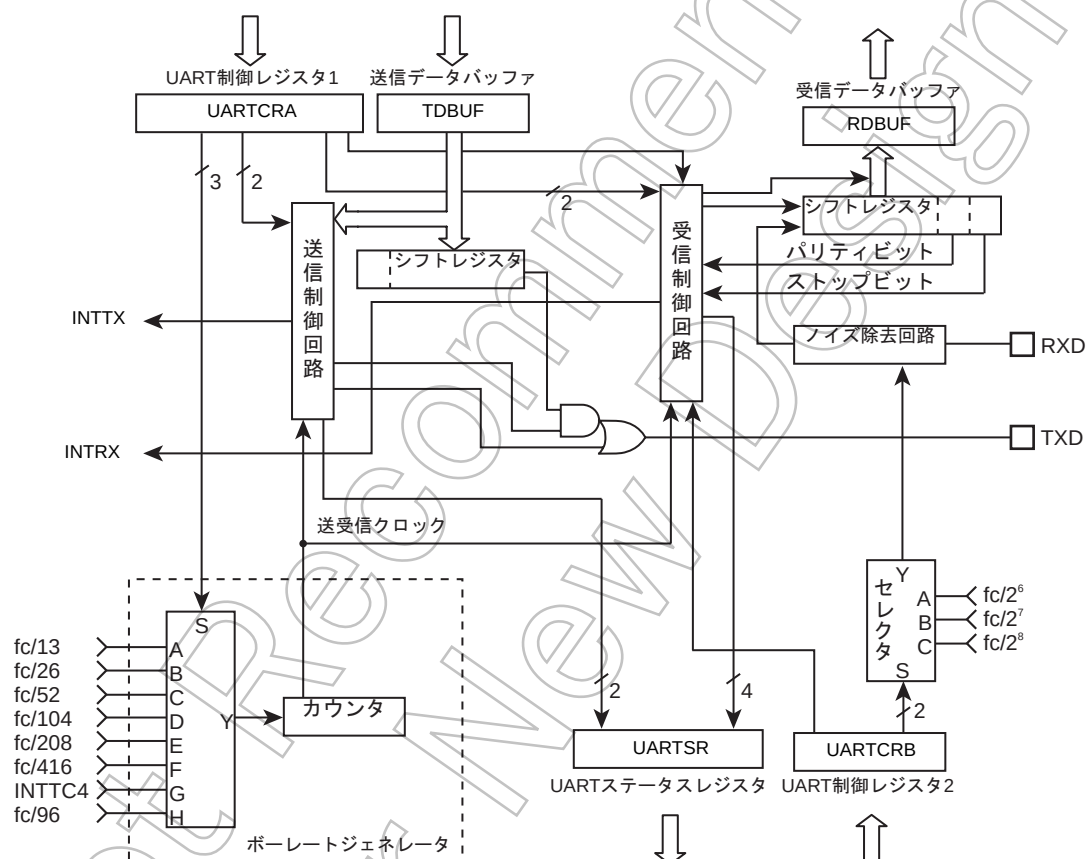
図 13-1 UART (非同期型シリアルインターフェース)
