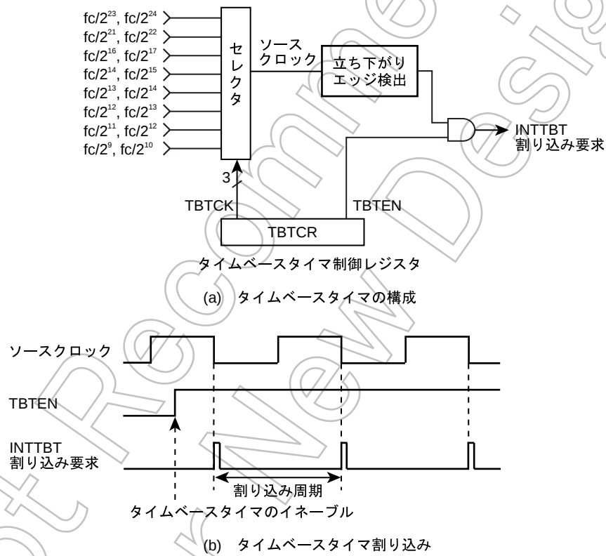
図 7-1 タイムベースタイマ
