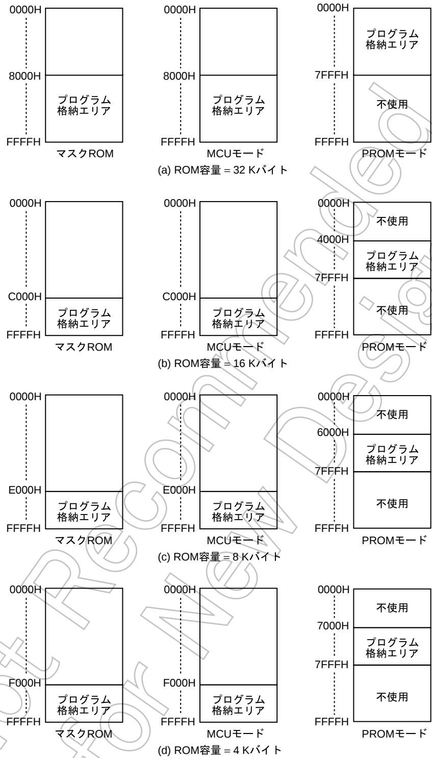
図 14-1 プログラム格納エリア
