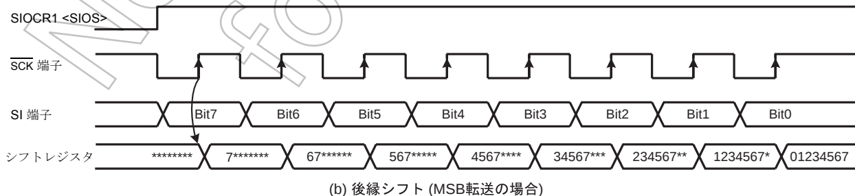
図 10-4 シフトエッジ
