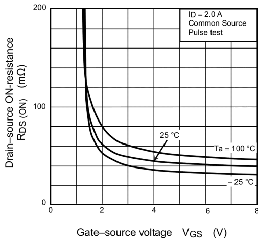
Fig. 7.3 R_{DS(ON)} - V_{GS}
