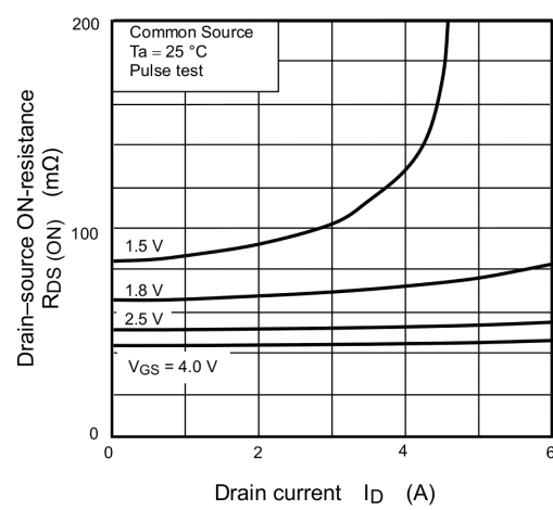
Fig. 7.4 R_{DS(ON)} - I_D
