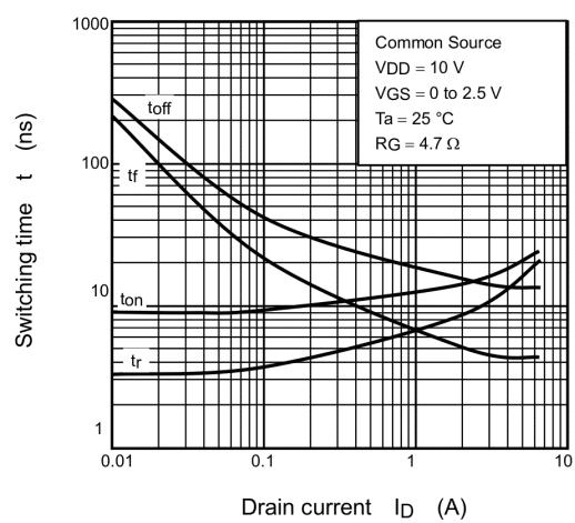
Fig. 7.10 t - I_D
