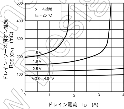
図 7.4 R_{DS(ON)} - I_D
