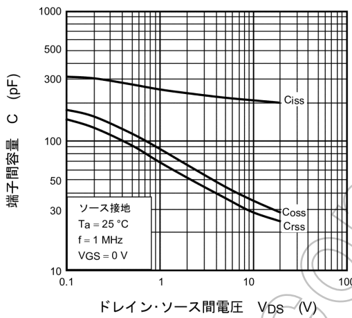
図 7.9 C - V_{DS}
