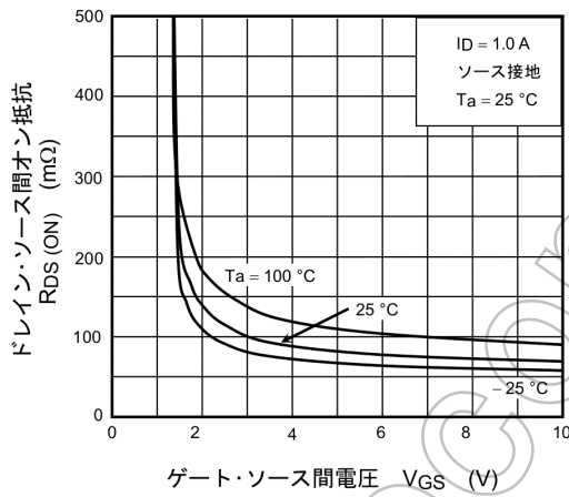
図 7.3 R_{DS(ON)} - V_{GS}
