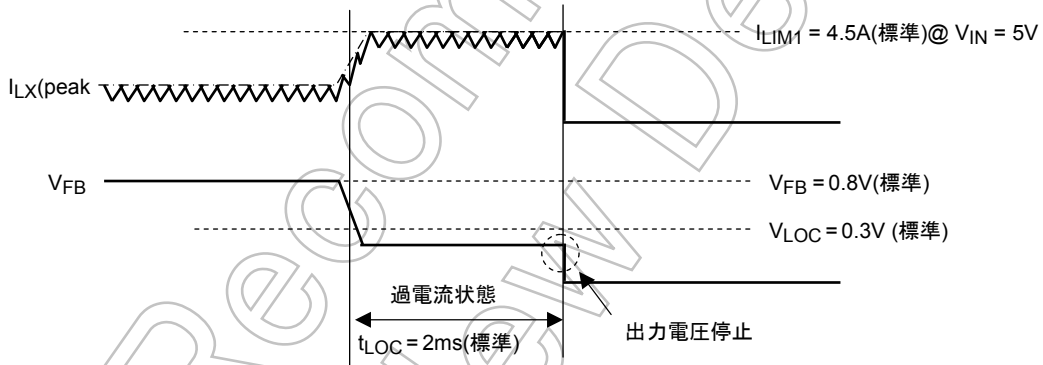
図 4 過電流保護動作
