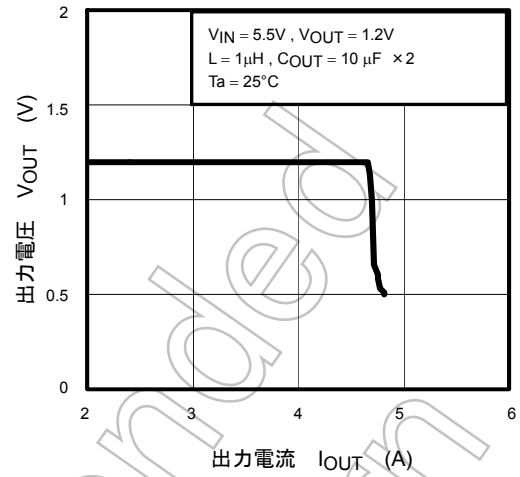
過電流特性
