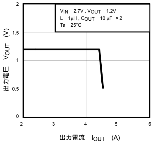
過電流特性
