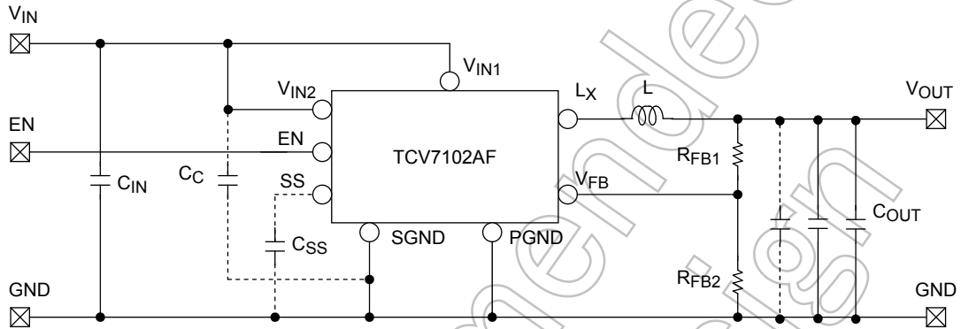
図 1 TCV7102AF 応用回路例
