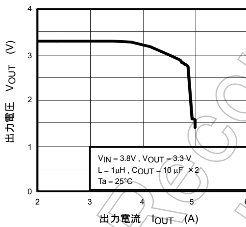
過電流特性
