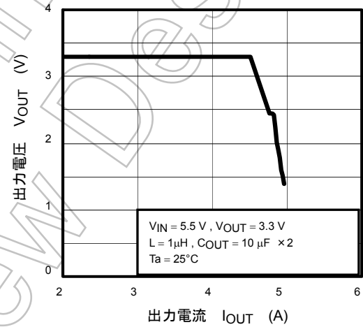
過電流特性
