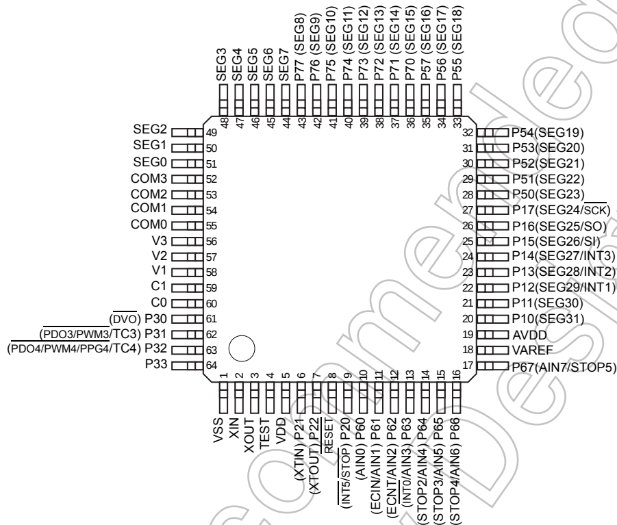
図 1-1 ピン配置図
