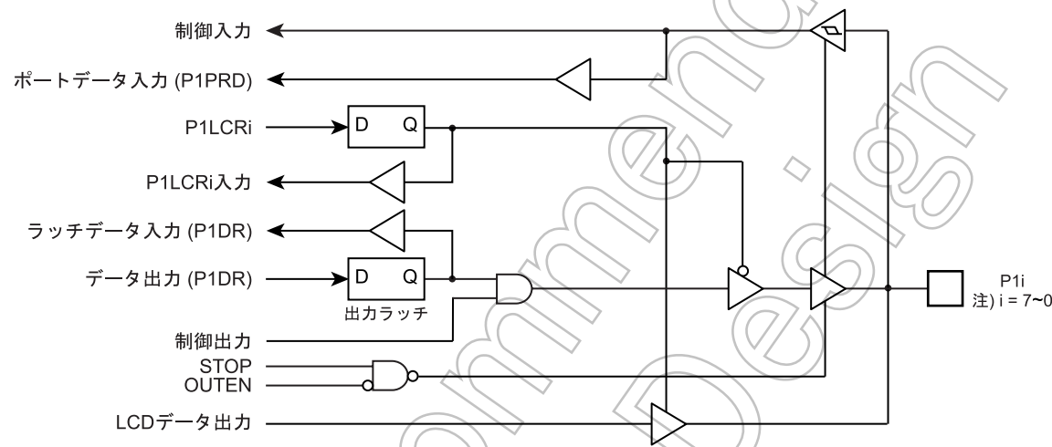
図 5-2 P1 ポート
