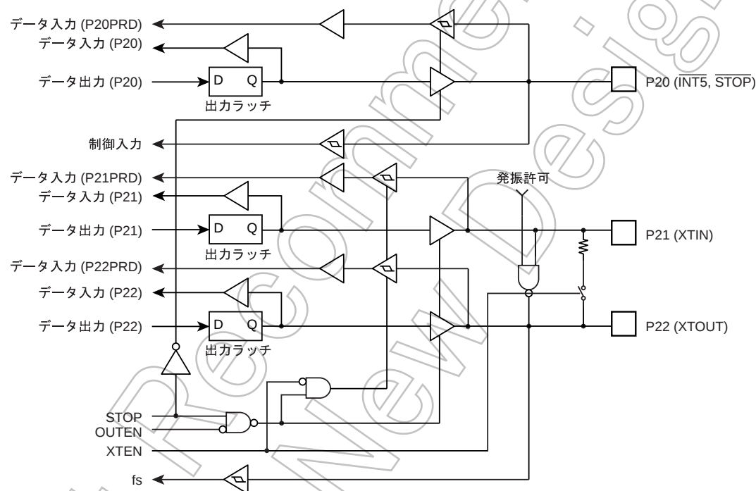
図 5-3 P2 ポート
