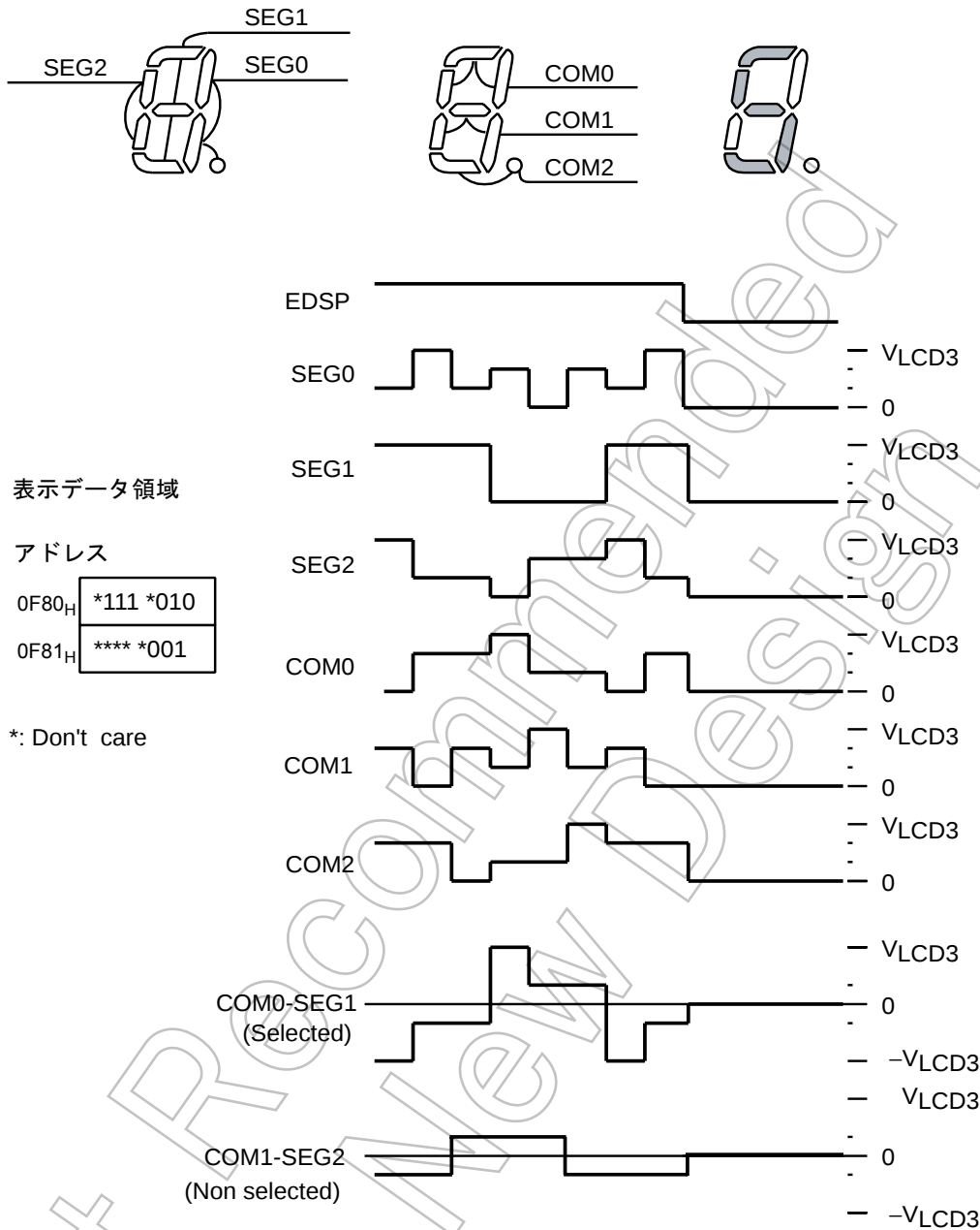
図 13-9 1/3 デューティ (1/3 バイアス) 駆動
