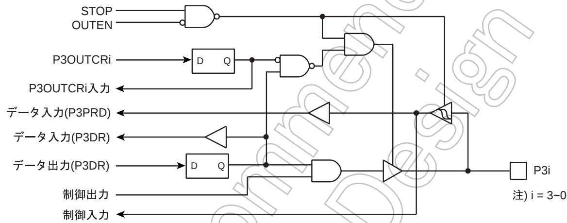
図 5-4 P3 ポート
