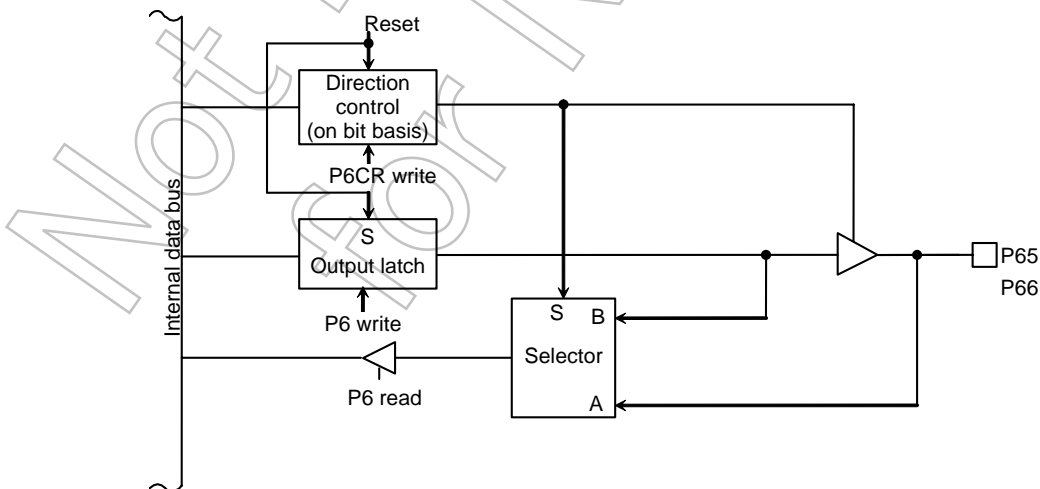
Figure 3.5.20 ポート 65, 66
