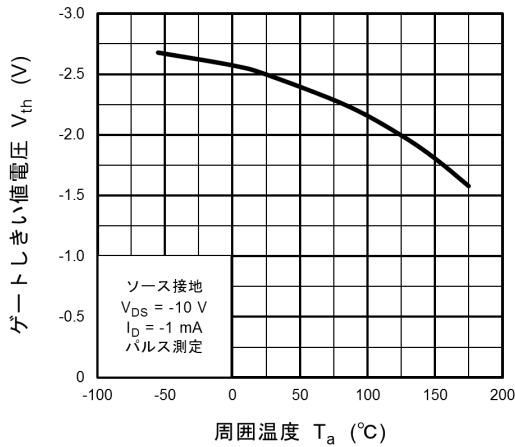
図 8.9 V_{th} - T_a
