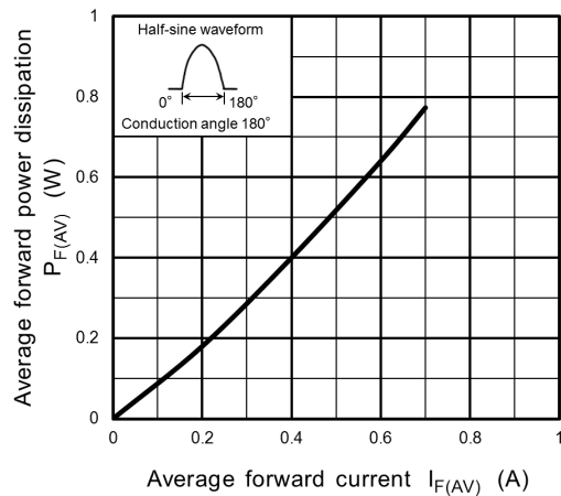
Fig. 10.2 P_{F(AV)} - I_{F(AV)}
