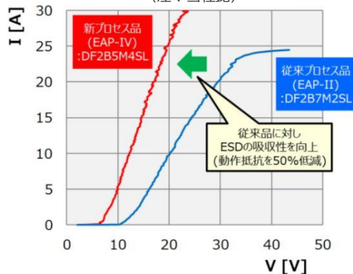
ESDパルス 吸収性能 (注：当社比)
