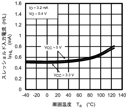
図 12.2.9 I_{FHL} - T_a
