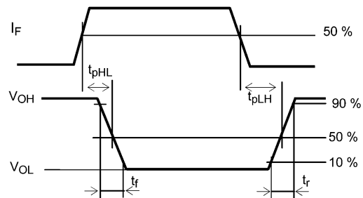
図 12.1.5 伝搬遅延時間測定回路, 波形
