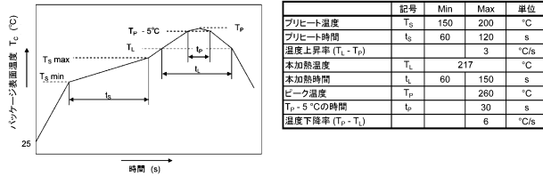
図 13.1.1 鉛フリーはんだ使用時の温度プロファイル一例
